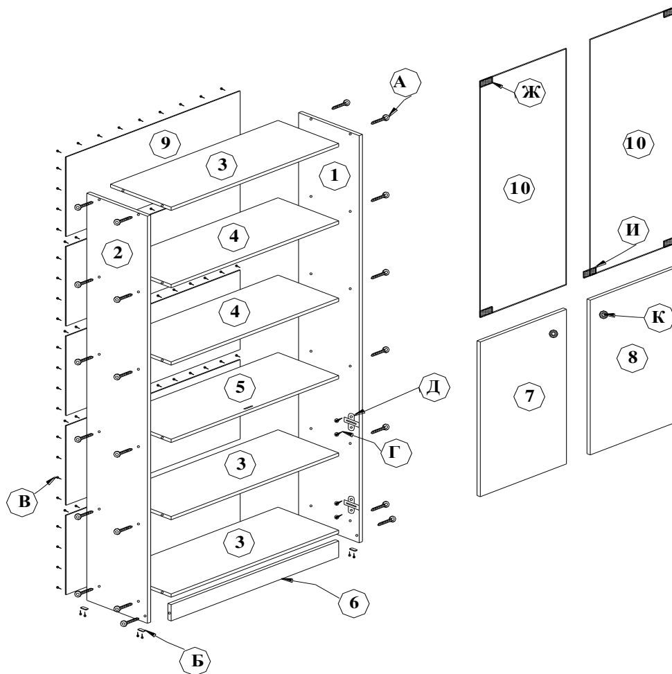
Ст-15 Стеллаж островной со стеклом 2000x850x300
